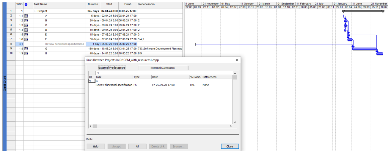
Рис. 32. Зв'язування окремого завдання з іншого проекту і діалогове вікно Зв'язки між проектами.
