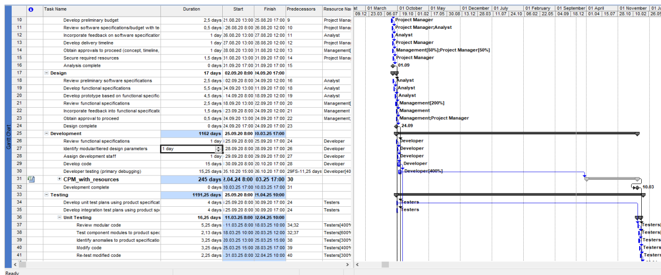
Рис. 29. Підпроект CPM with resources у проекті Software development plan. Реалізована вставка на деякому рівні WBS головного проекту.
